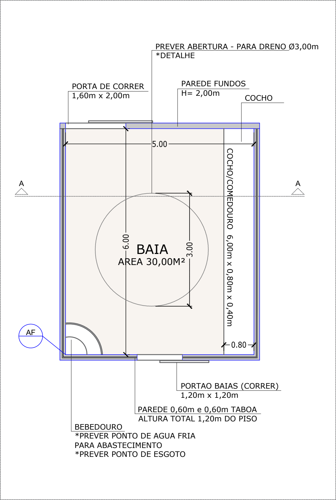
DETALHE BAIA
