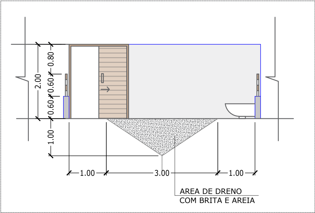
CORTE AA DETALHE PARA DRENO
